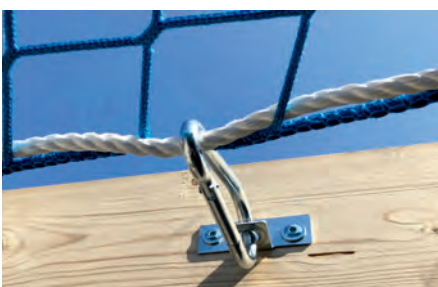
Abb. 5: Befestigungsmöglichkeit für kleinformatige Schutznetze: LUX-Top Ben Schutznetzhalter (Foto: ST QUADRAT Fall Protection S.A)
