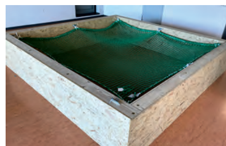
Abb. 2: Kleinformatiges Schutznetz ca. 3 m x 3 m in einem Holzrahmen (Foto: BG BAU – T.-P. Glaser)
