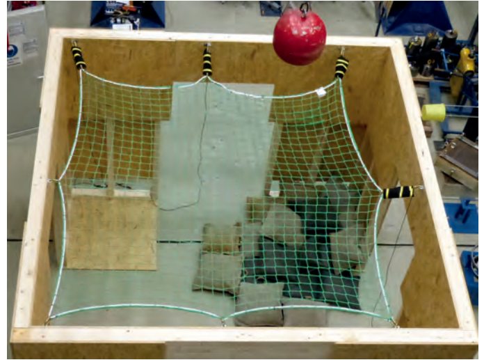
Abb. 4: Versuchsvorrichtung zum Prüfen eines kleinformatigen Schutznetzes mit den Maßen 3 m x 3 m (Foto: BG BAU – T.-P. Glaser)
