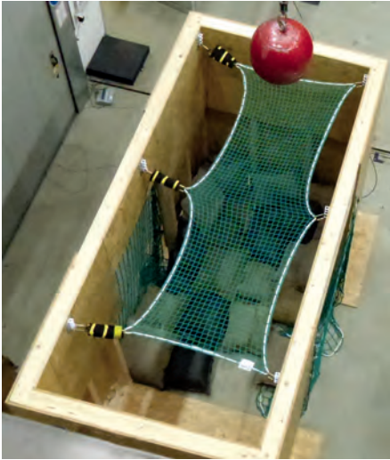
Abb. 3: Versuchsvorrichtung zum Prüfen eines kleinformatigen Schutznetzes mit den Maßen 1 m x 3 m (Foto: BG BAU – T.-P. Glaser)
