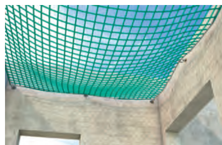
Abb. 1: Kleinformatiges Schutznetz ca. 3 m x 2,50 m in einer Treppenhausöffnung (Quelle: H.ZWEI.S GmbH)
