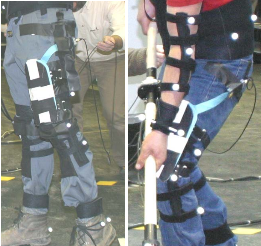
Abbildung 2.9: Druckmesspad zur Messung der Auflagekräfte der Schaufel am Oberschenkel (links); Abstützung des Schaufelstiels beim Schaufeln auf dem Oberschenkel (rechts)
