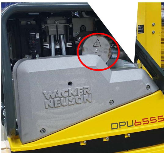
Abb. 8: Rüttelplatte mit Dieselpartikelfilter
