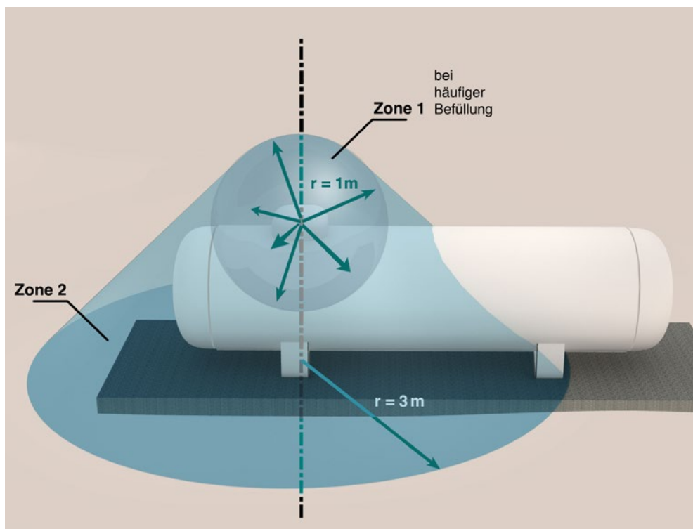
Abb. 15 Geometrische Abmessungen der Zone eines ortsfesten Druckgasbehälters im Freien (Verzicht auf Darstellung von Druckregleinrichtung, Rohrleitung und Verbrauchseinrichtung)
