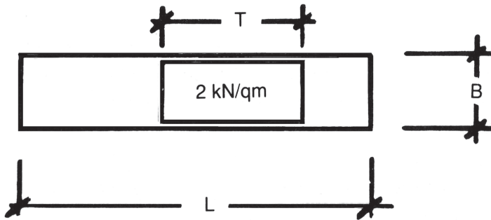
Grundriss des Personenaufnahmemittels
