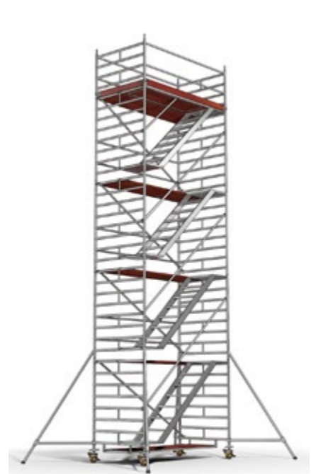
Abb. 49 Fahrbare Arbeitsbühne mit Treppenaufstieg und Abstützungen
