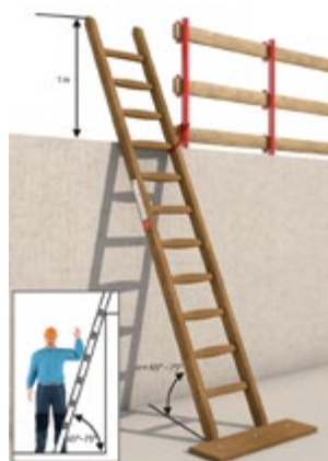
Abb. 42 Sicherung gegen Wegrutschen
