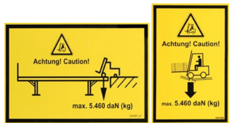
Abb. 21 Kennzeichnung der maximalen Achslast zur Befahrbarkeit von Wechselbehältern mit Gabelstaplern
