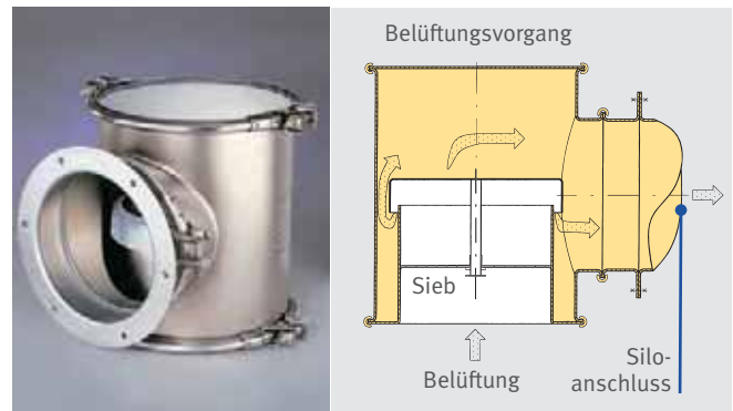
Abb. 6.24 und 6.25 Belüftungsventil
