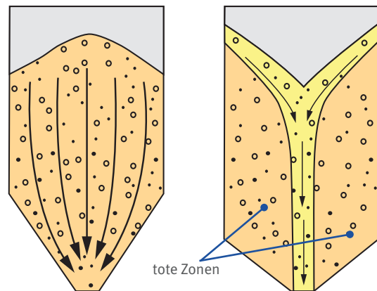
Abb. 4.2 links: Massenfluss, rechts: Kernfluss
