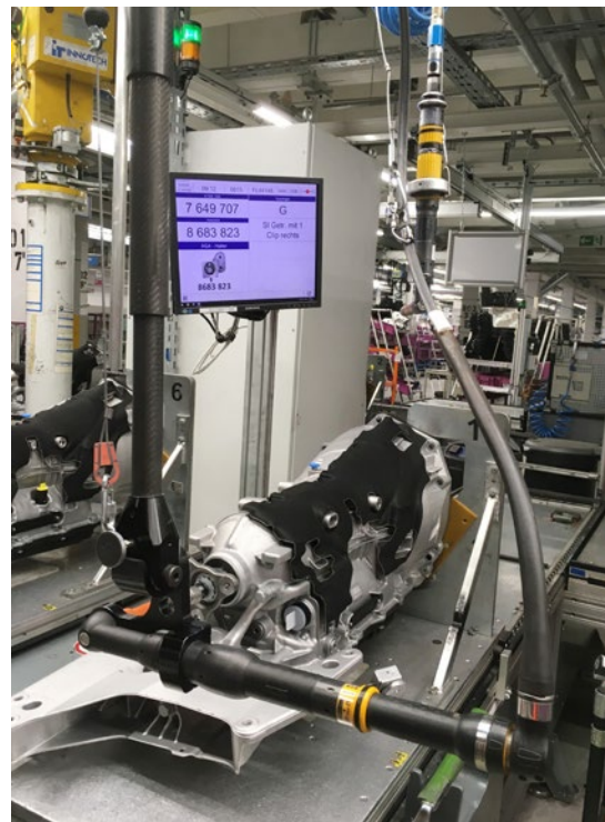
Abb. 27 Ersatz von Schlagschrauben durch Drehmomentschrauber. Die Benutzung von Gehörschutz ist nicht notwendig. Balancer verbessern die Ergonomie.
