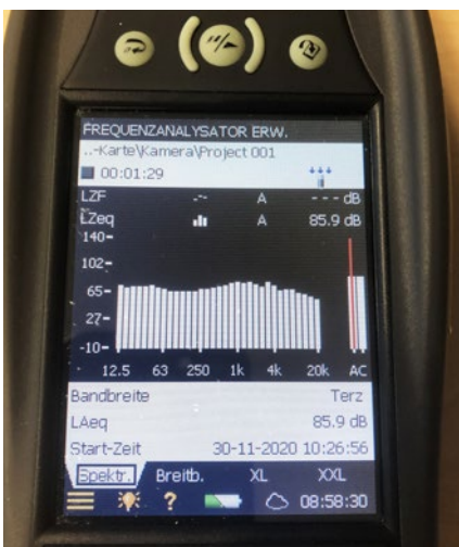
Abb. 22 Terz-Frequenzanalyse mit der Software des Messgeräts
