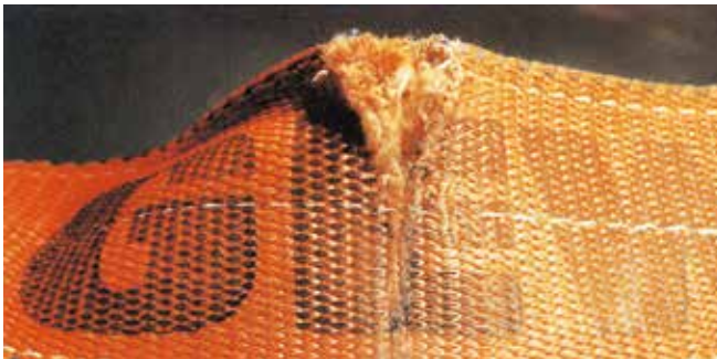
Bild 23-14: Durch scharfkantige Last eingeschnittenes Hebebänder
