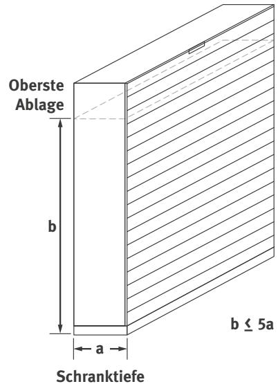
Abb. 5 b Höhen-Tiefen-Verhältnis für Schränke mit Schiebe- oder Rolllüren
