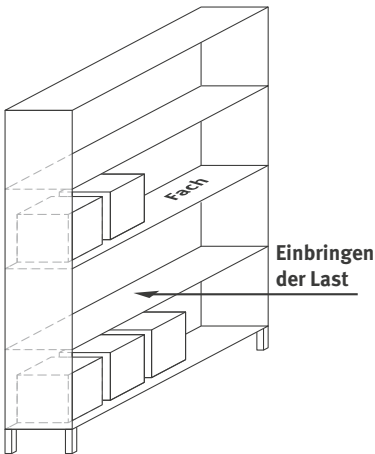
Abb. 8a 4 Fächer = Feld eines Einfachregal
