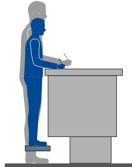
Typ 6 Steh-Arbeitsplatz nicht höhenverstellbar (Tisch- höhe angepasst an das 95. Perzentil)
