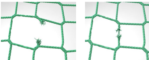
Abb. 9 Sichtprüfung des Netzes (Anmerkung: Linke kleine Abbildung zeigt zerstörte Maschen, rechte kleine Abbildung den Abrieb an der Masche)
